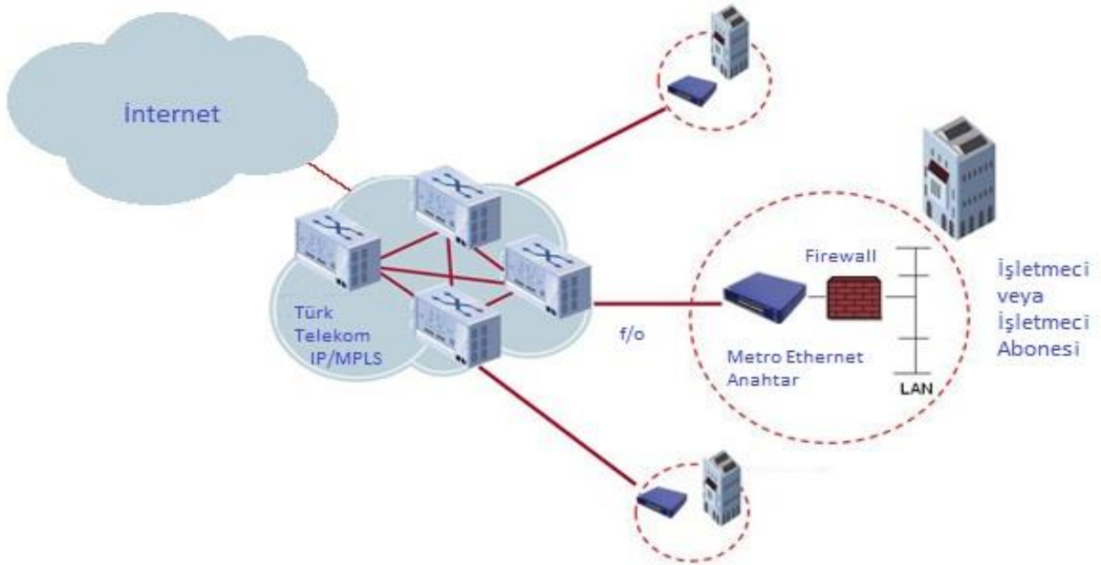
Şekil-2: Al-Sat Yöntemine Göre ME İnternet Topolojisi
