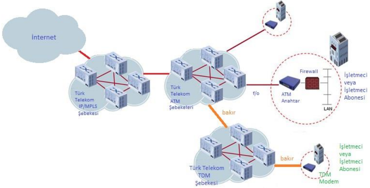
Şekil-1: Al-Sat Yöntemine Göre ATM/FR İnternet Topolojisi
