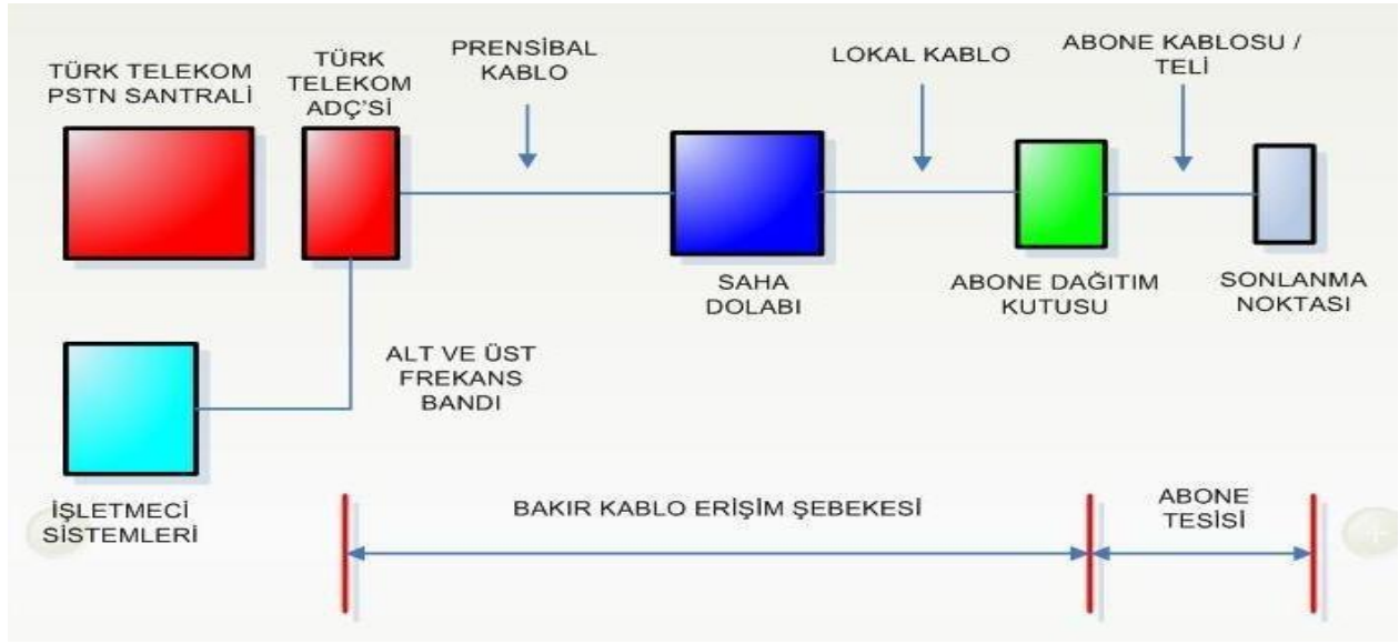
ŞEKİL-2b: Yerel Ağa Ayrıştırılmış Tam Erişim Hizmetine ilişkin Ortak Yerleşim Planı
