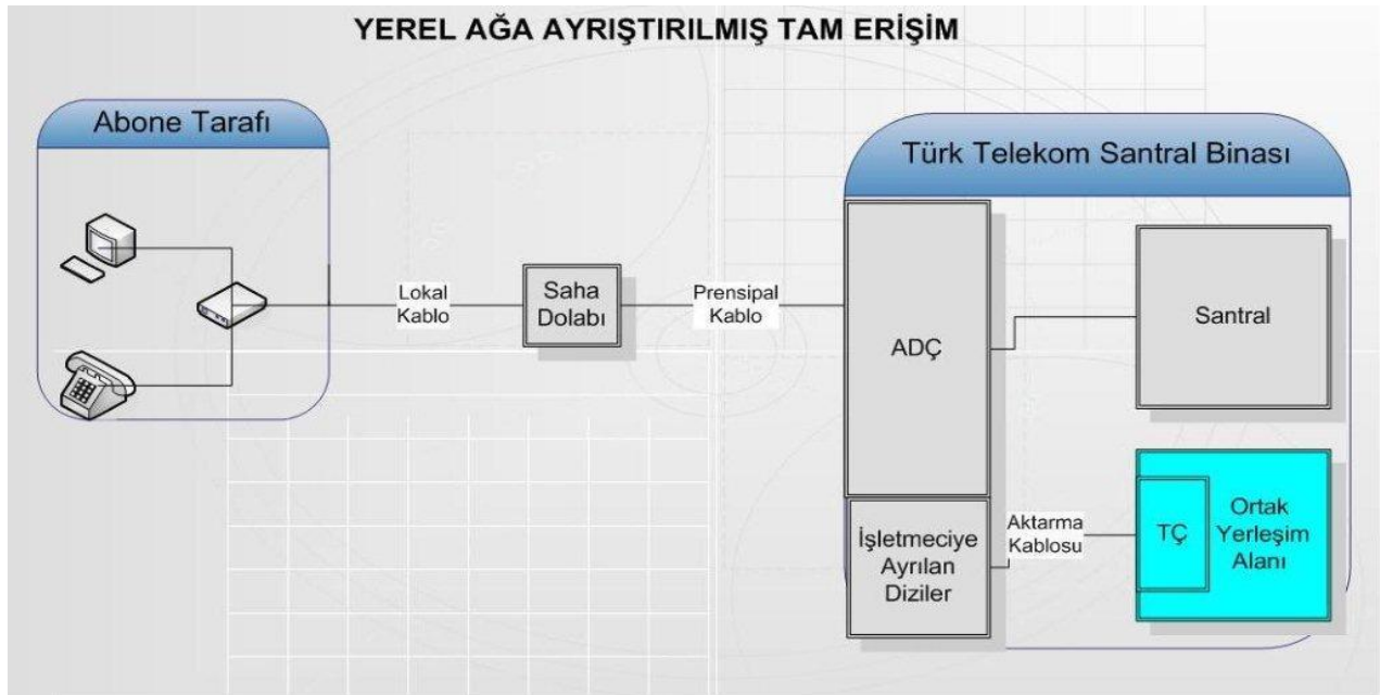
ŞEKİL-2b: Yerel Ağa Ayrıştırılmış Tam Erişim Hizmetine ilişkin Ortak Yerleşim Planı
