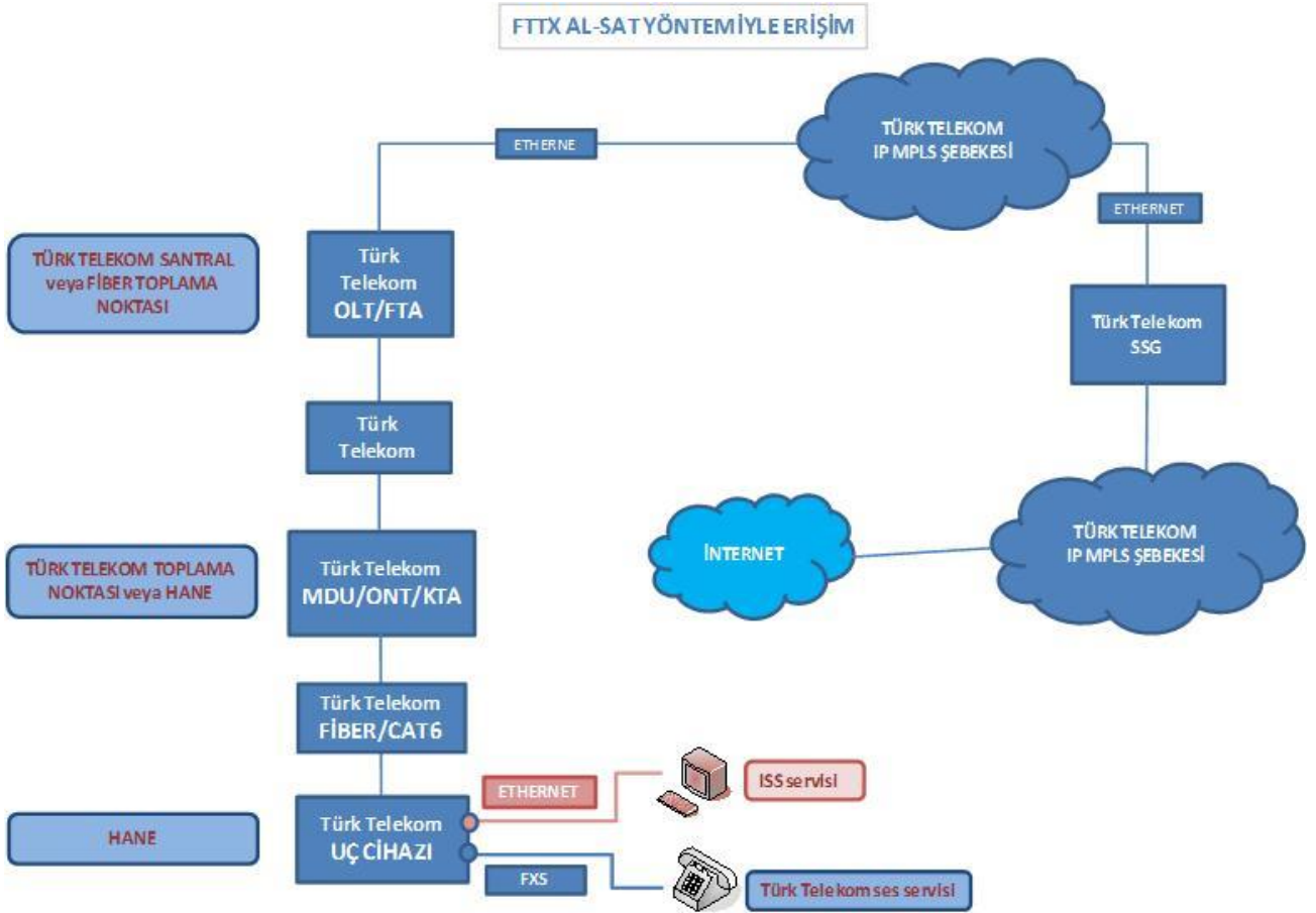
Şekil-1 İşletmeciler için Al-Sat Yöntemiyle FTTx Versiyon 1 Toptan Satış Hizmeti’ne Göre Topoloji
